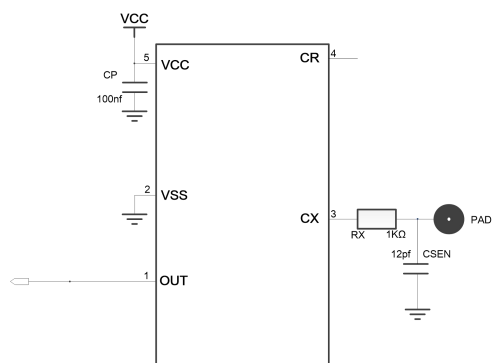
简化原理图
