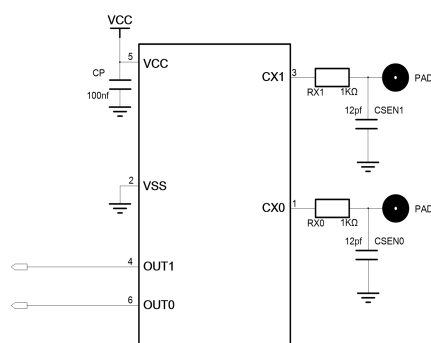
简化原理图
