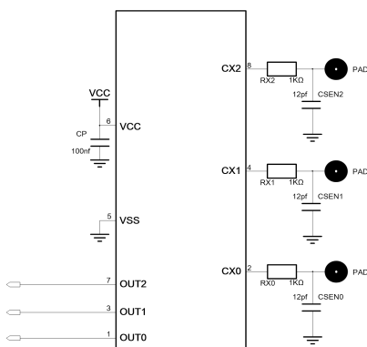
简化原理图
